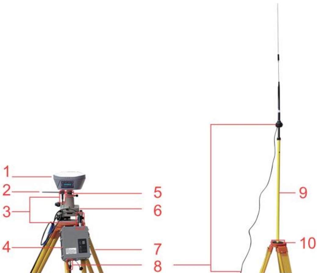
Рисунок 4.3 Базовая станция с внешним радиомодемом
