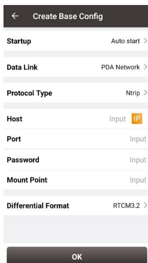
Рисунок 4.6 Базовая конфигурация – Сеть контроллера (Ntrip)
